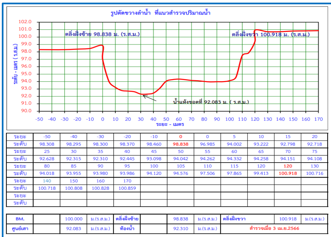
รูปที่ 7-9 จัดทำรูปตัดขวางลำน้ำ สถานี ห้วยแม่ป่าไผ่ สะพานบ้านตีนตก ต.นาคอเรือ อ.ฮอด จ.เชียงใหม่ (ท้ายโครงการอ่างเก็บน้ำ ห้วยแม่ป่าไผ่ อันเนื่องมาจากพระราชดำริ จังหวัดเชียงใหม่)
