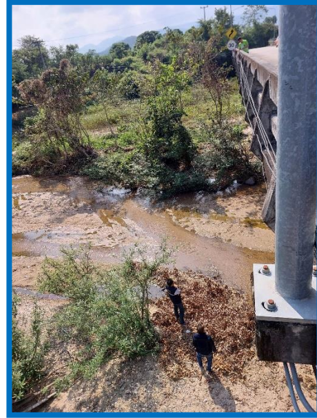
รูปที่ 7-9 จัดทำรูปตัดขวางลำน้ำ สถานี ห้วยแม่ป่าไผ่ สะพานบ้านตีนตก ต.นาคอเรือ อ.ฮอด จ.เชียงใหม่ (ท้ายโครงการอ่างเก็บน้ำ ห้วยแม่ป่าไผ่ อันเนื่องมาจากพระราชดำริ จังหวัดเชียงใหม่)
